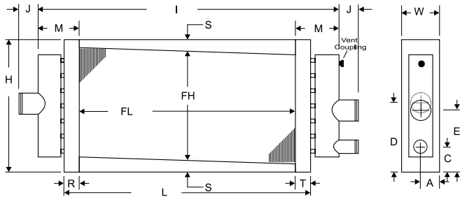
Figure 4 - DA, LA Dimension Info
